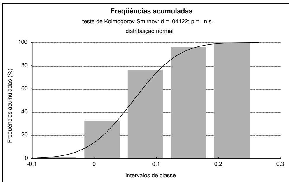
Figura 10. Percentuais acumulados de freqüência relativa dos dados experimentais comparados à curva normal hipotética.
